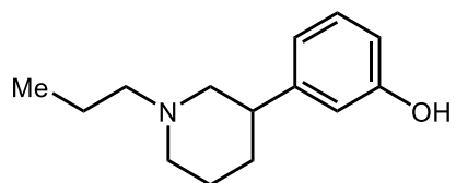
Preclamol (3-PPP)
